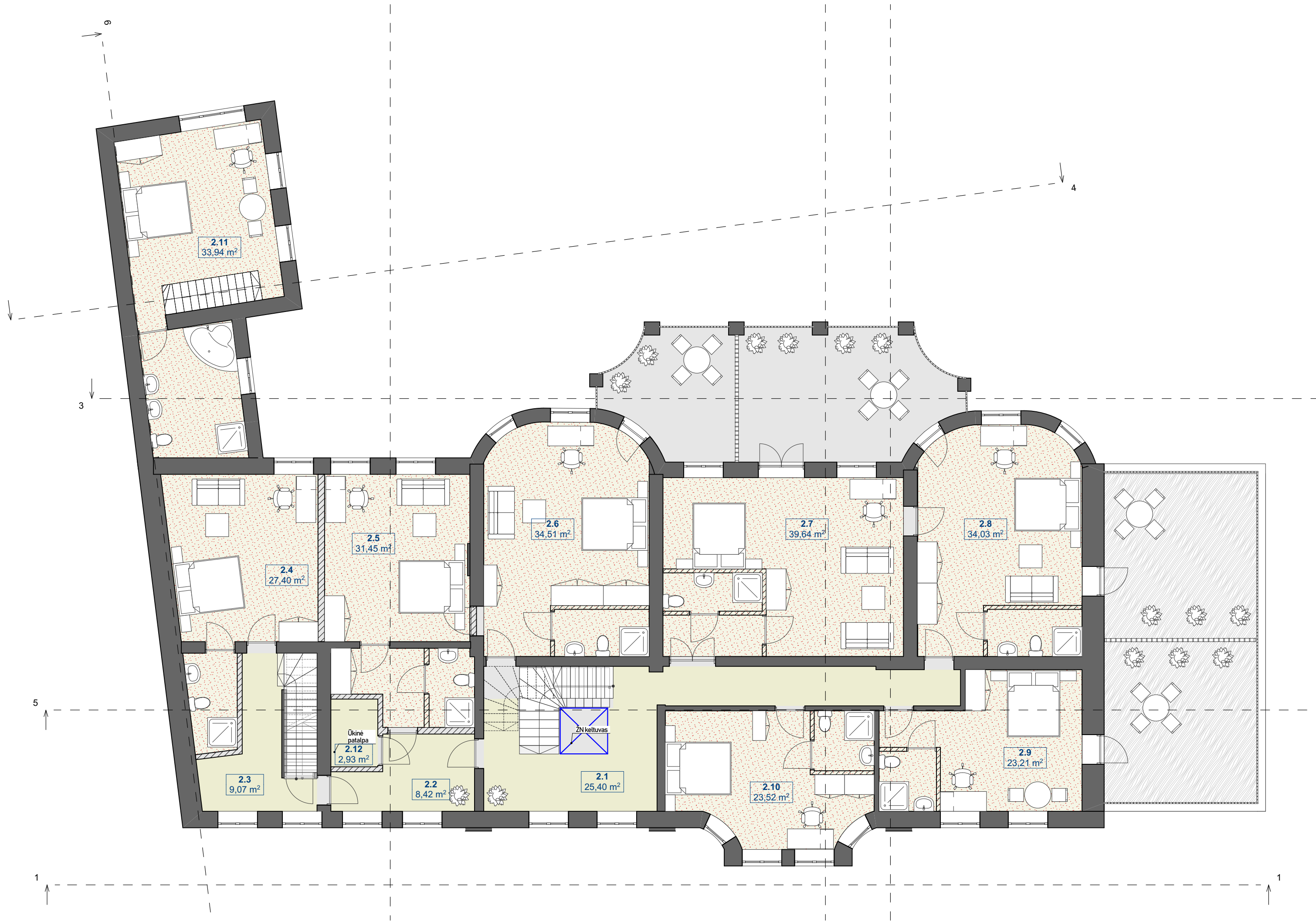
1:100 ANTRAS AUKŠTAS
